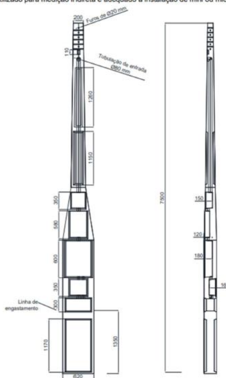
Imagem 2: poste padrão C6
